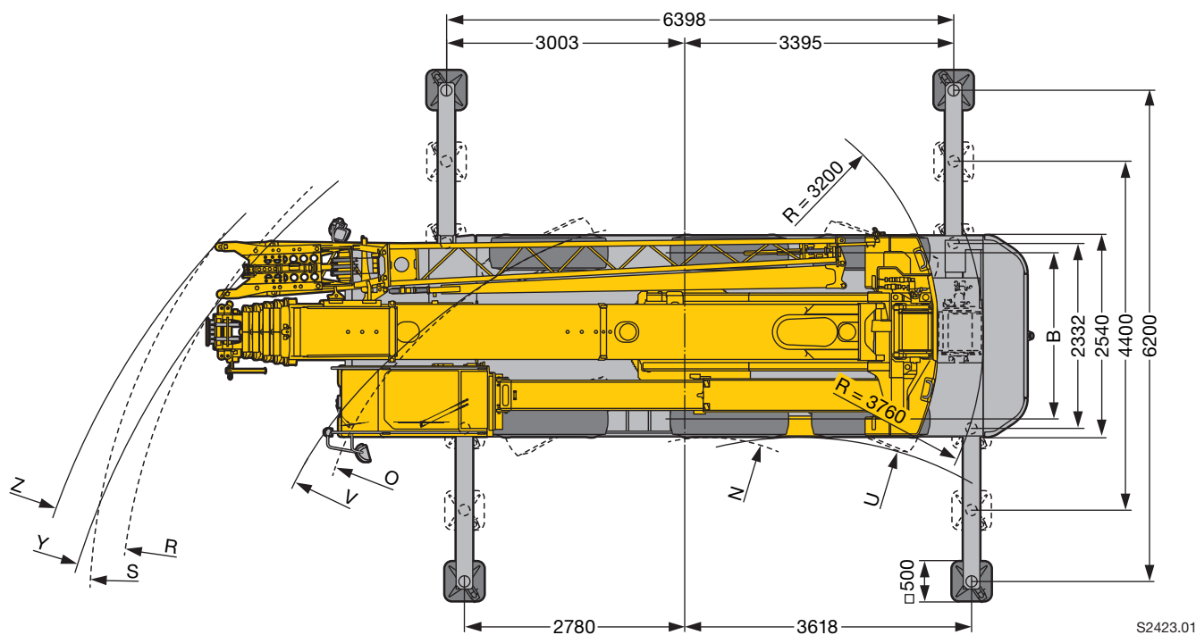
Maße · Dimensions · Encombrement · Dimensioni · Dimensiones · Размеры mm
